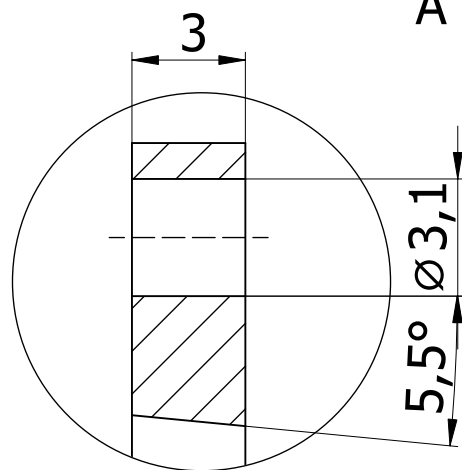
Detail Z 5:1
